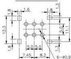
P.C.B HOLE DETAIL
