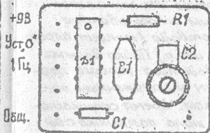
Вид со стороны р./деталей Вид со стороны печ. проводн.
