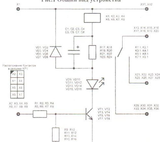
Рис.2 Схема электрическая принципиальная одного канала Описание работы модуля
