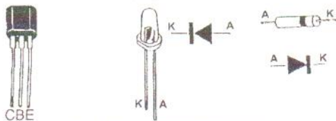
Рис.4 Цоколевка элементов
