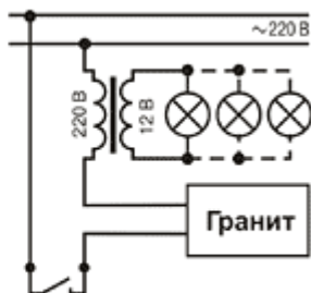
Рис. 2 (для ламп на 12 В)
